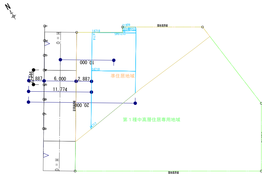
天空率-道路斜線 配置図 (適合建物) S = 1 : 200
