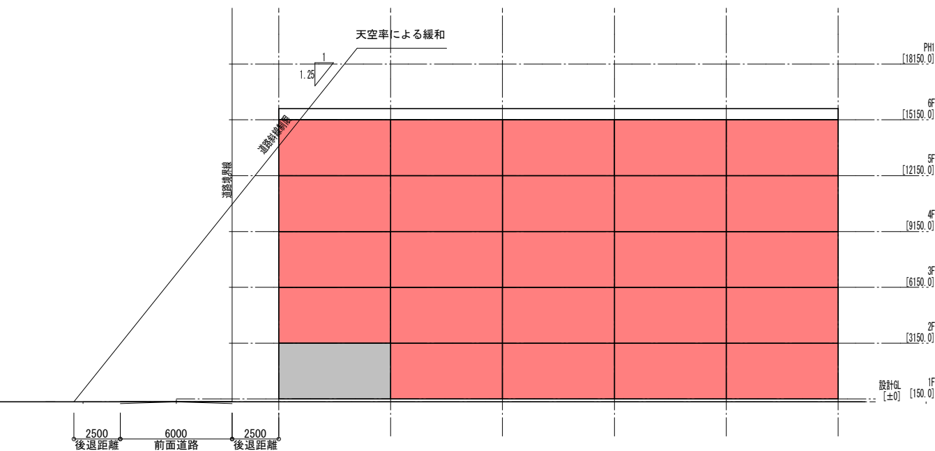
道路斜線制限
